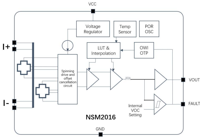
Figure 1. NSM2016 功能框图
