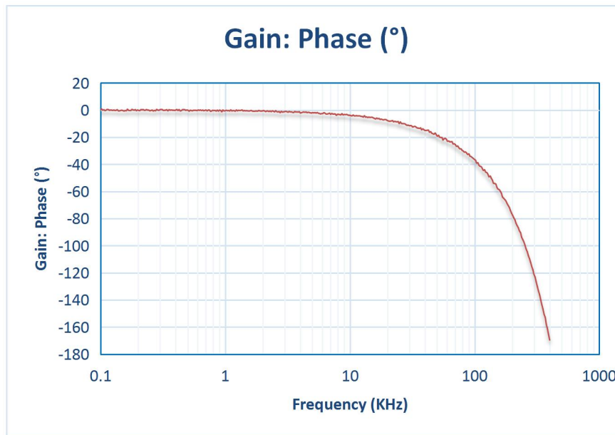
Figure 6.4 NSM2016 相频响应曲线
