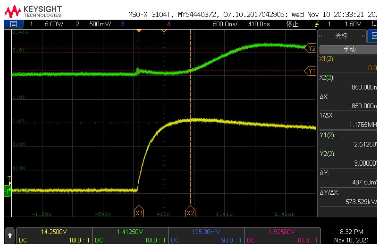
(3) 延迟时间/Propagation Delay time 黄色：原边电流、绿色：VOUT
