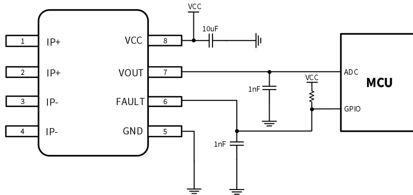
Figure 7.1 NSM2016 典型应用电路
