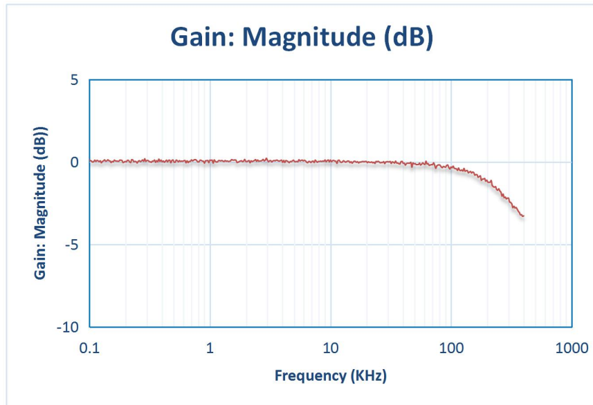
Figure 6.3 NSM2016 幅频响应曲线
