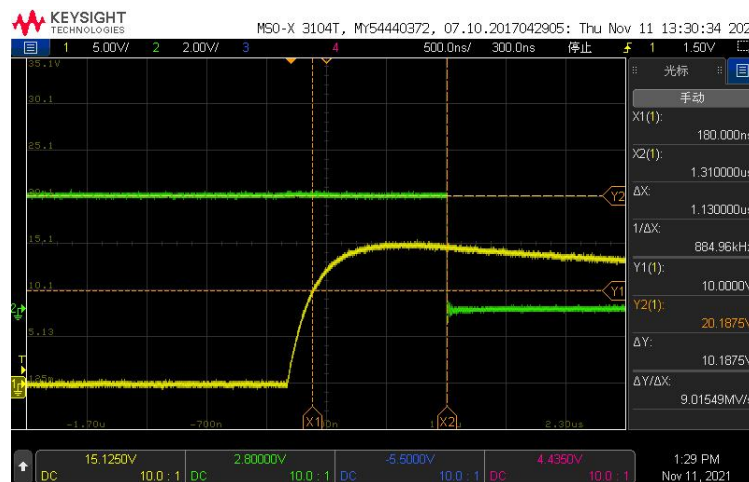
(4) Fault 响应时间 黄色：原边电流、绿色：Fault
