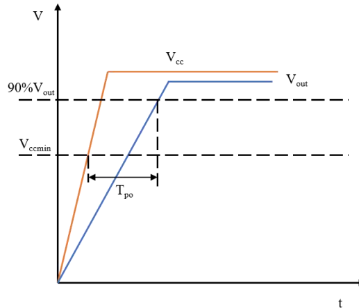
Figure 6.5 NSM2016 上电时间定义
