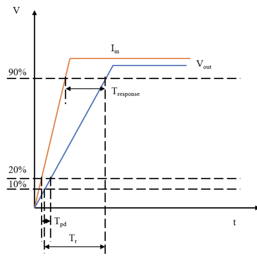
Figure 6.6 NSM2016 响应时间定义
