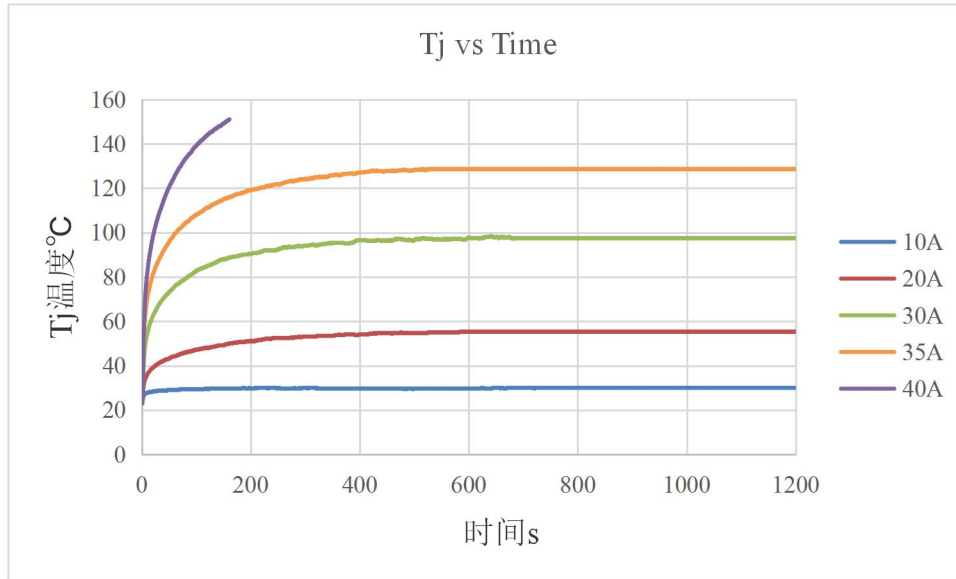
Figure 7.3 NSM2016 在不同电流下结温曲线
