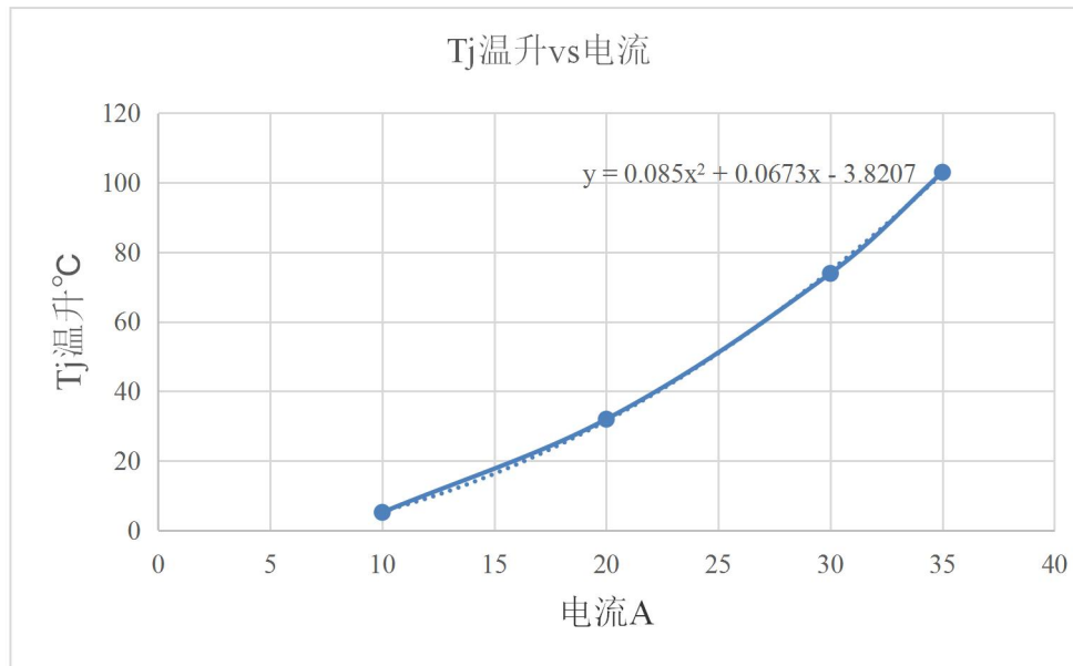
Figure 7.4 NSM2016 在不同电流下结温曲线预估函数(PCB 在 worst case)
