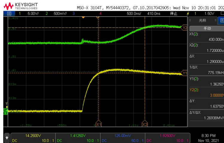
(2) 响应时间/Response time 黄色：原边电流、绿色：VOUT
